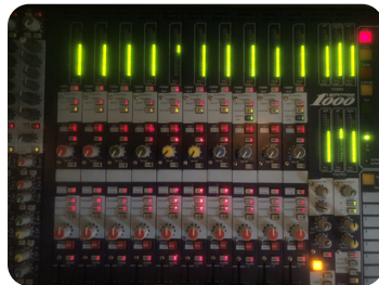
Panne de bargraphe
