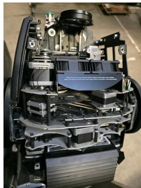
Remise en état Martin Mac 700/550
